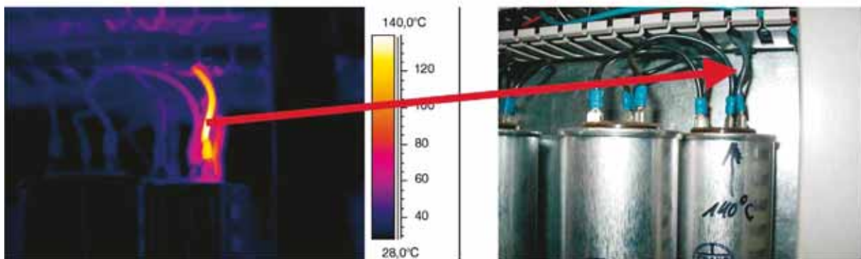
Defekter Steckkontakt
